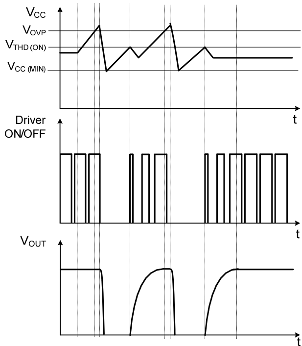
Fig.7 OVP Case
