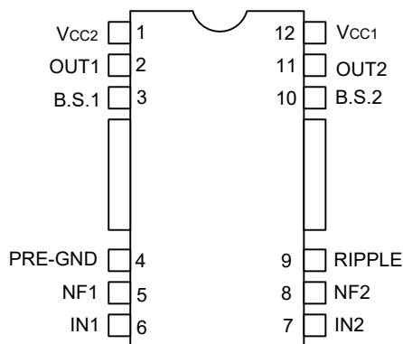
DIP-12H
