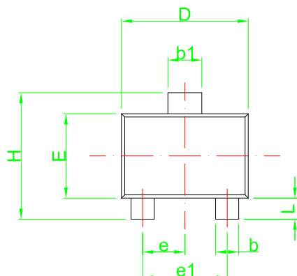
TOP SIDE
