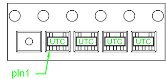
SOT-23-5 T/R
