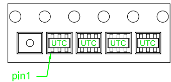
SOT-23-6 T/R
